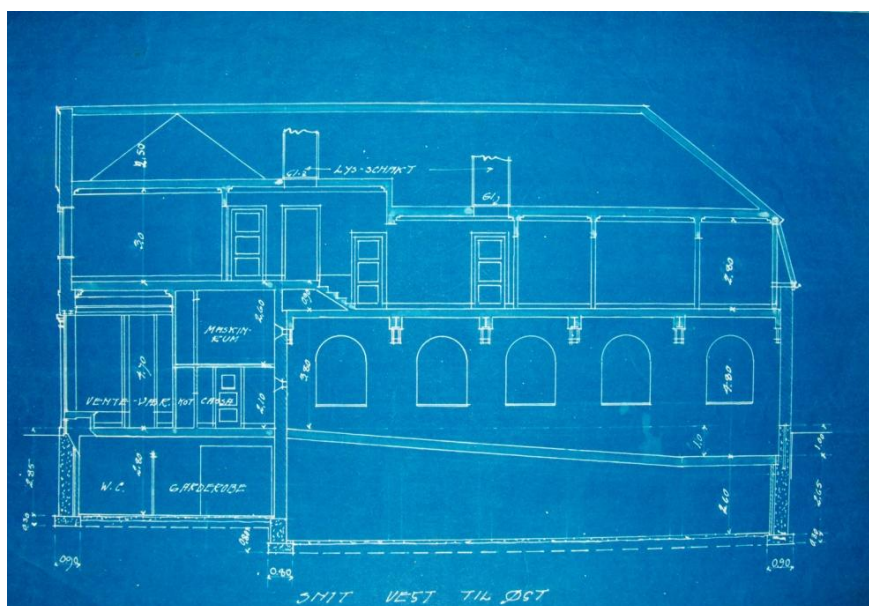
III 9.3: Tverrsnitt gjennom bygget, som viser vestibyle og billettluke samt salens lengde og skråning.
