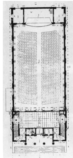
Kino-Palæets grunnplan over hovedetasjen.
