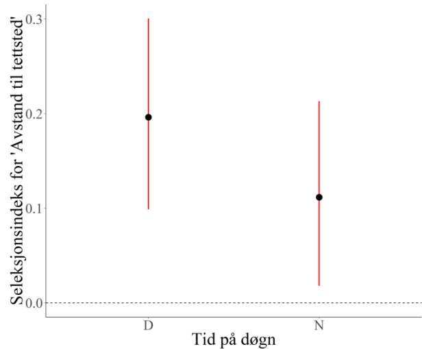
Figur 6: Seleksjonsindeks for avstand til tettsted i forhold til tid på døgn, modellert for ulv i Skandinavia (gjennomsnitt og 95% konfidensintervall). D = dag og N = natt. Den stiplede linjen ved y = 0 indikerer ingen seleksjon, verdier > 0 viser seleksjon for større avstander, og < 0 for mindre avstander til tettsted enn forventet fra tilgjengelig habitat.
