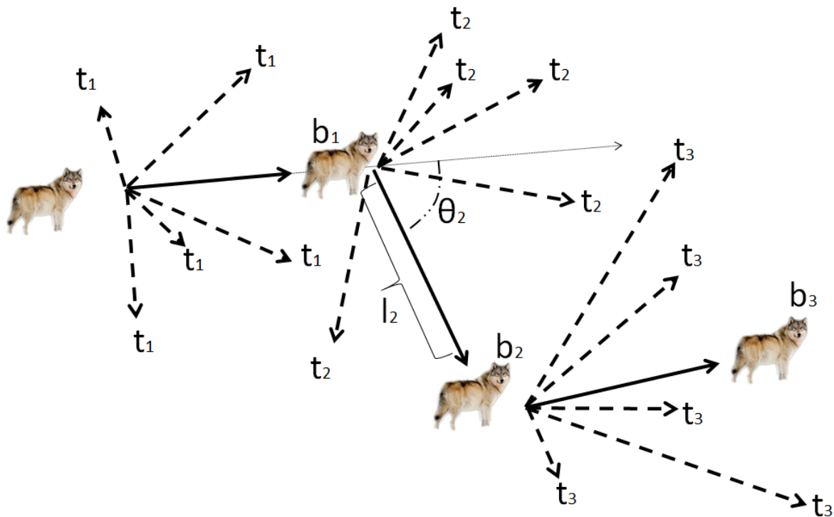
Figur 3: Skjematisk forklaring av stegvalganalysen SSF. Heltrukne piler viser ulvens reelle steg. Alle reelle steglengder ( l ) og retninger ( \vartheta ) ble brukt til å lage en fordeling av lengder og retninger (Figur 4). Fra disse fordelingene trakk vi for hvert reelt steg 5 tilfeldige steg (stiplede piler). Til slutt sammenlignet vi habitatet ved de brukte ( b ) og tilfeldige ( t ) endepunktene for hvert steg.
