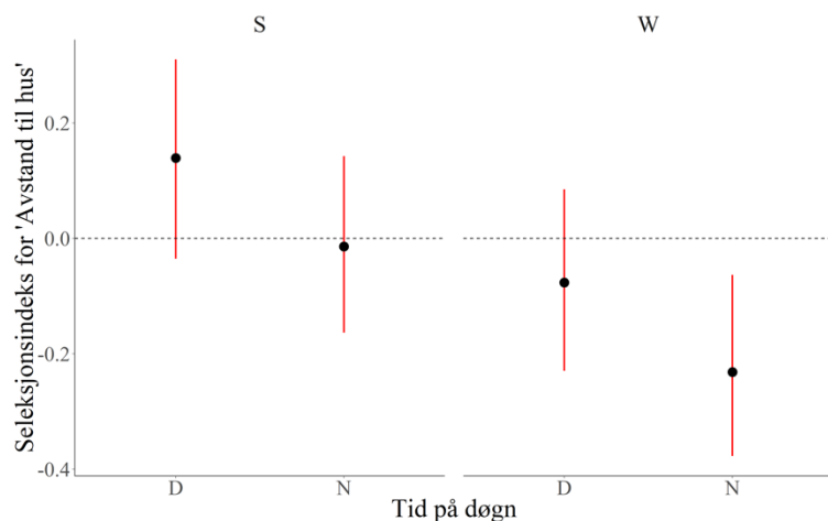
Figur 10: Seleksjonsindeks for avstand til bebodde hus i forhold til årstid og tid på døgn, modellert for ulv i Norge (gjennomsnitt og 95% konfidensintervall). D = dag, N = natt, S=sommer, W = vinter. Den stiplede linjen ved y = 0 indikerer ingen seleksjon, verdier > 0 viser seleksjon for større avstander, og < 0 for mindre avstander til hus enn forventet fra tilgjengelig habitat.
